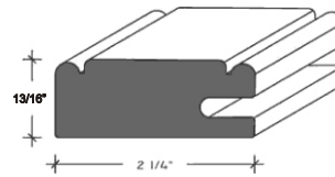
2 1/4" Door Profile
